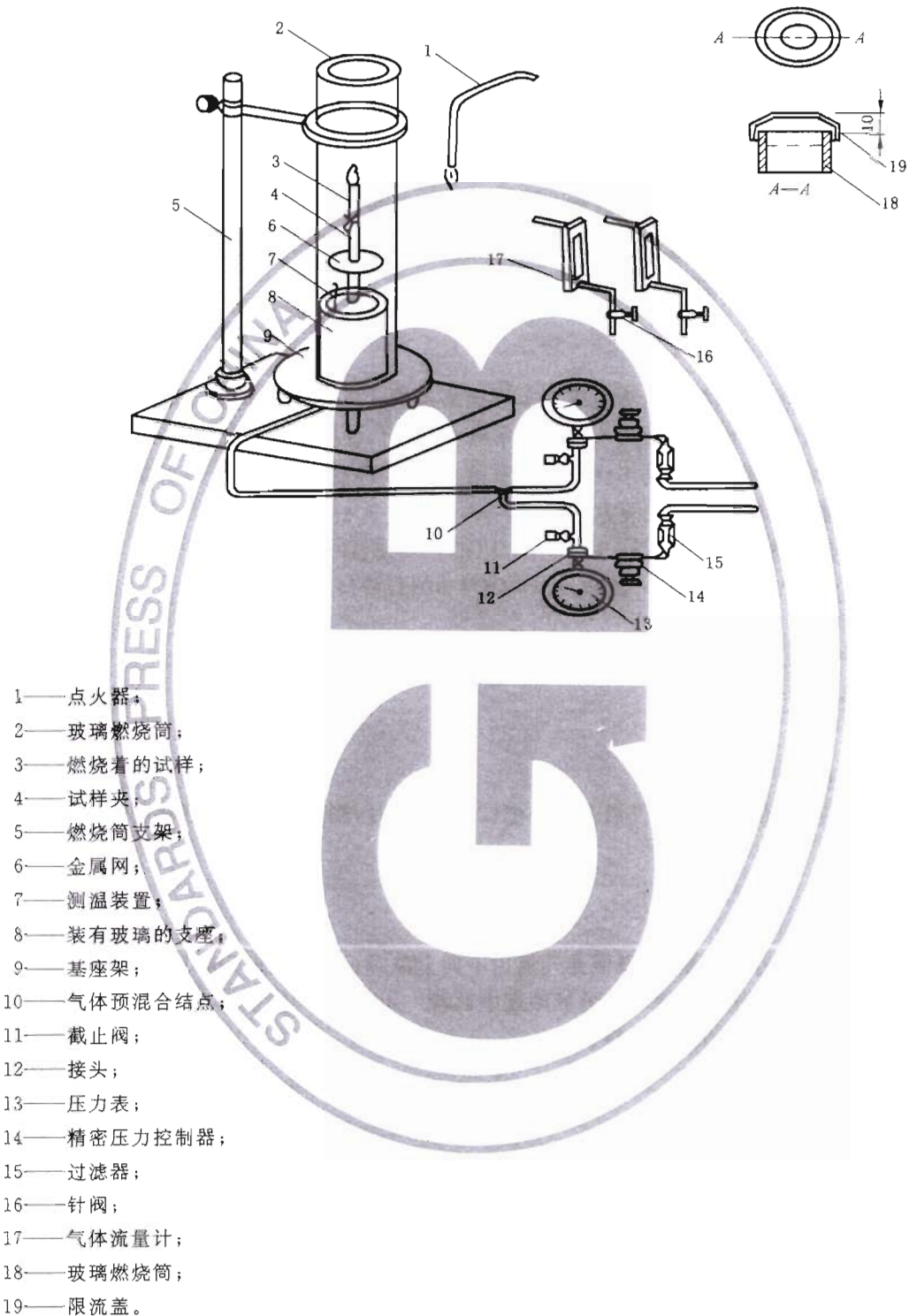
图 1 氧指数测定仪示意图
